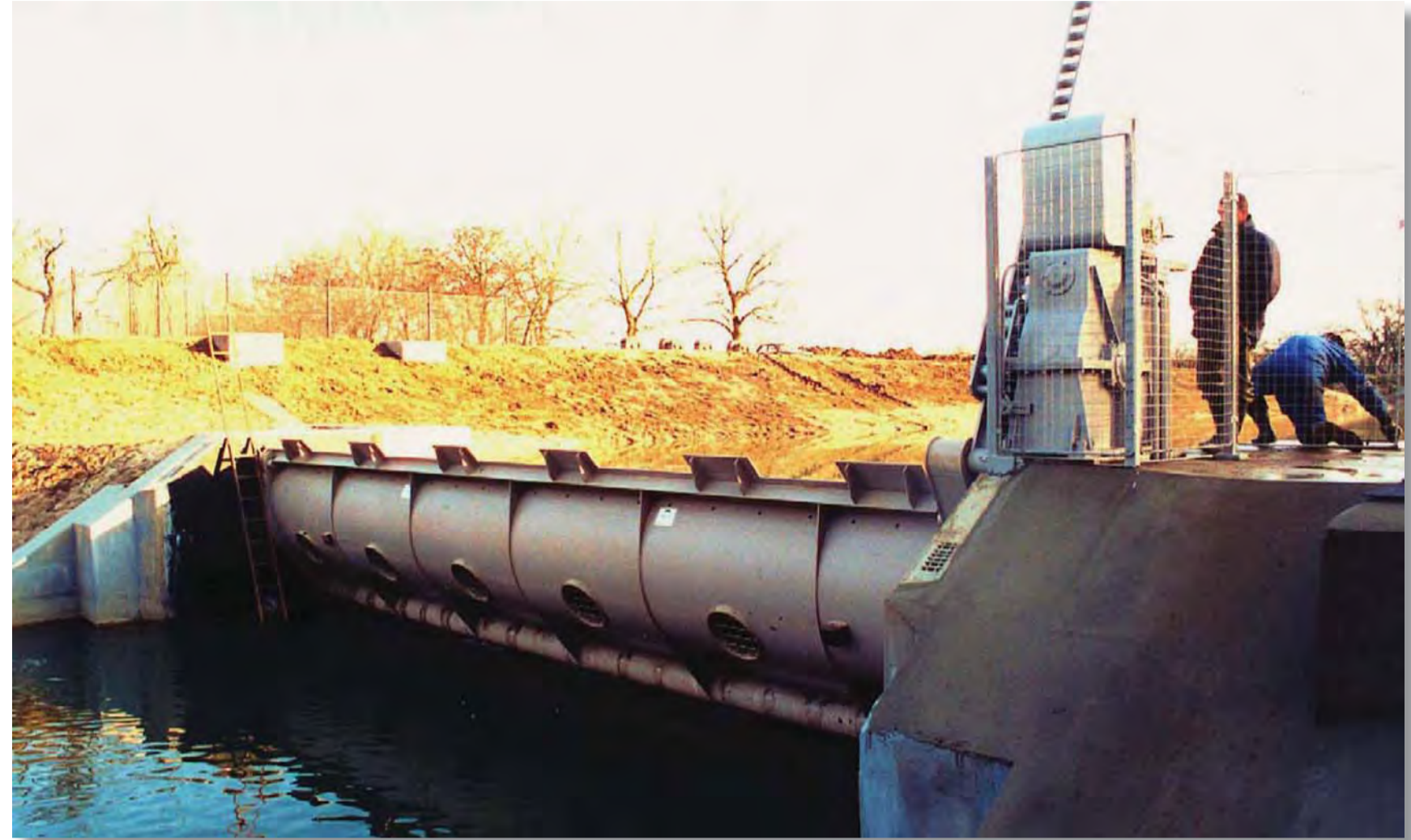
Jezová klapka Velička (Česká republika) Tilting gate Velička (Czech Republic) Клапан платины Величка (ЧР)
